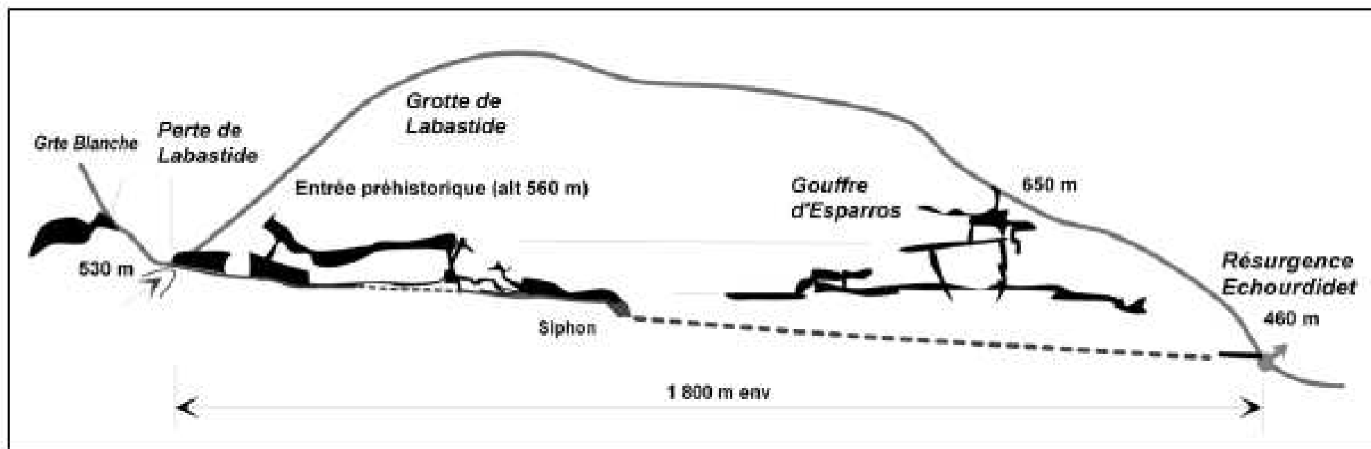
Coupe. Illustration JP. CASSOU 02 / 2009
